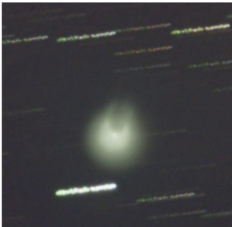
Podivně vypadající hlava komety 12P/Pons-Brooks po ourburstu 20. července 2023. Foto: Juan lacruz.
